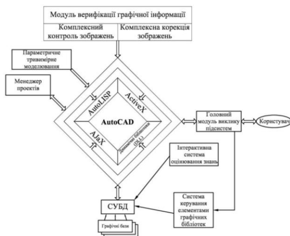
Рис. 1. Функціональна взаємодія модулів універсальної автоматизованої інформаційної системи
